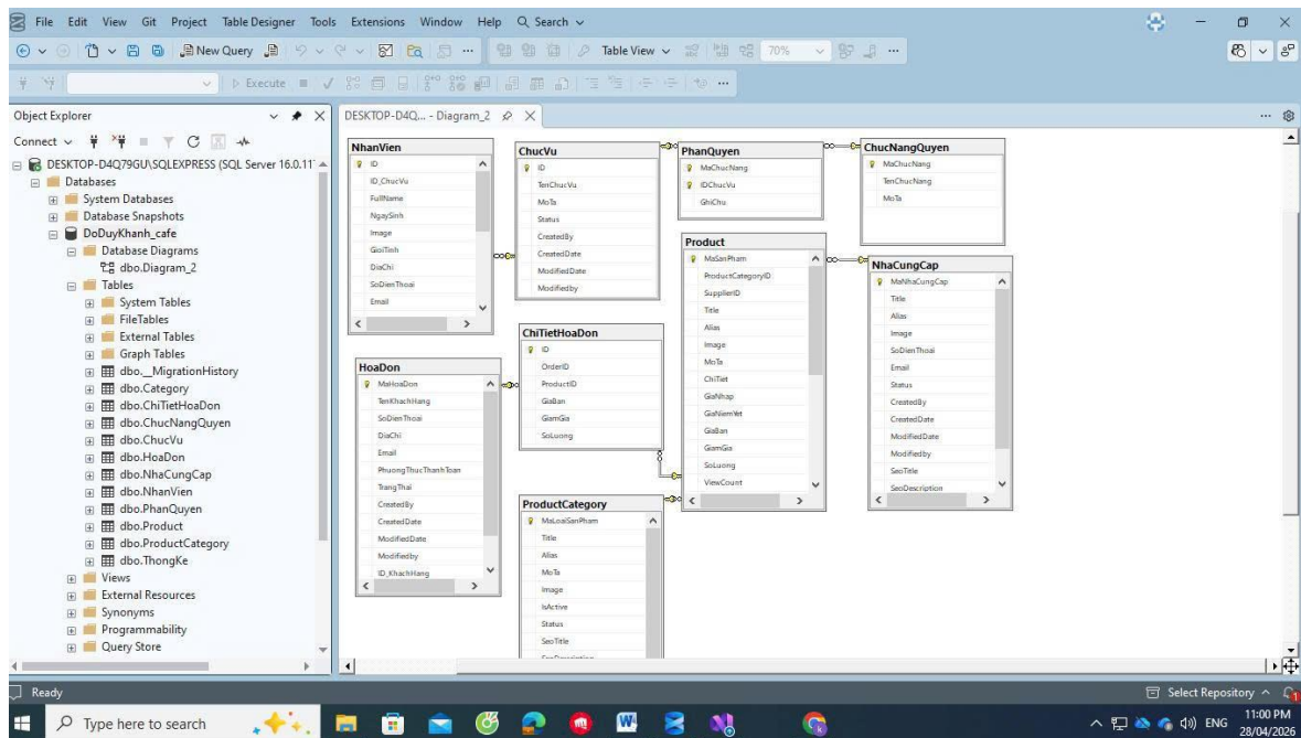
Hình 1. Sơ đồ logic được thiết kế bằng SQL Server
